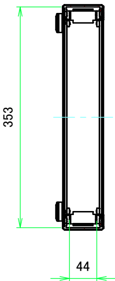
A-A ( 1:6 )
